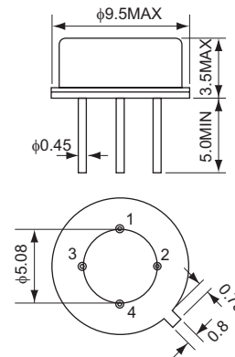
D04 / TO-39
